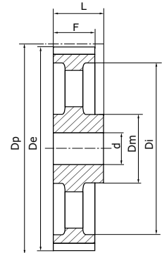
Typ 2E Hohl-Riemenscheibe
