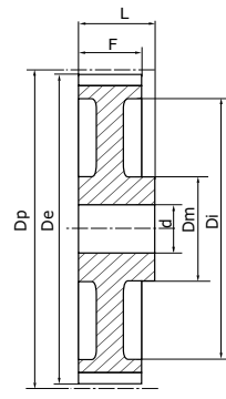
Typ 2A leichtere RiemenSchleibe
