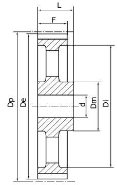
Typ 2E Hohl-RiemenSchleibe
