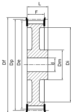
Typ 2AF leichtere Riemenleibe
