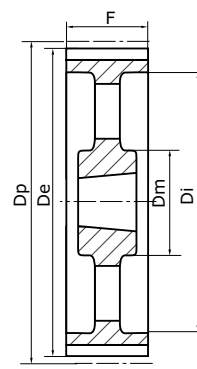
Typ 9E Hohl-Riemenscheibe
