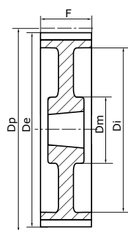
Typ 9A leichtere Riemenhleibe
