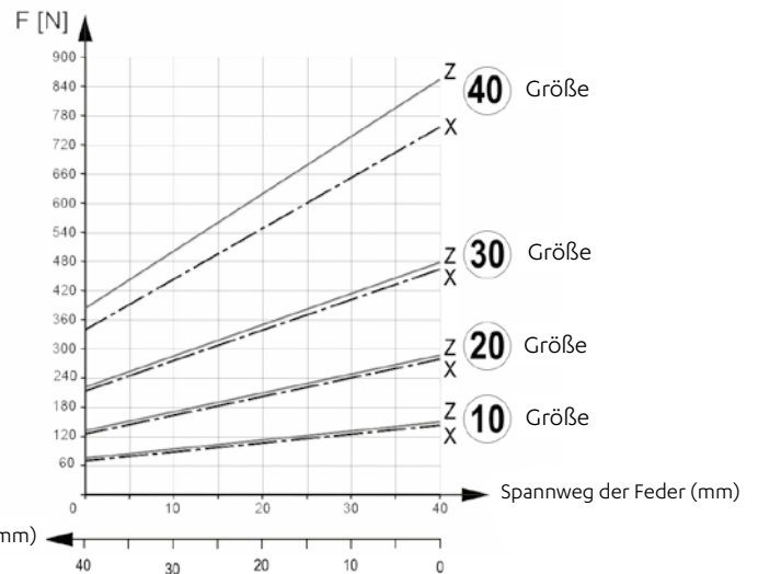
Belastungsdiagramm
