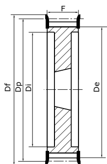
Typ 5F Vollschleibe mit Bordschleiben
