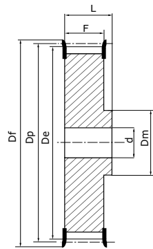
Typ 2F Vollscheibe mit Bordscheibe
