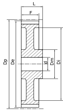
Typ 2A leichtere Riemenleibe
