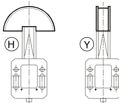
Positionierung der Kettengleiter
