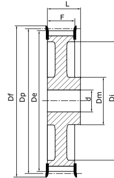
Typ 2AF leichtere RiemenSchleibe
