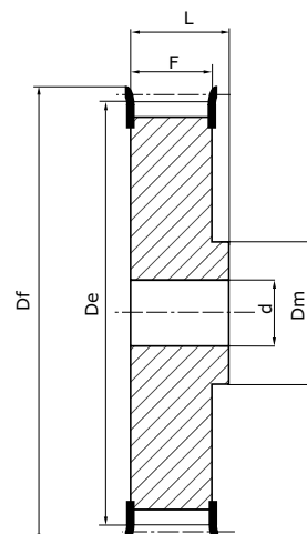
Typ 2F Vollscheibe mit Bordscheiben
