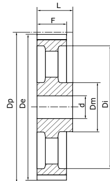
Typ 2E Hohl-Riemscheibe
