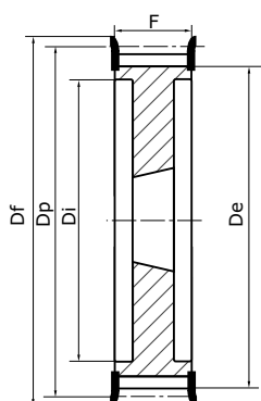
Typ 5F Vollscheibe mit Bordscheiben
