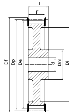
Typ 2AF leichtere Riemenscheibe
