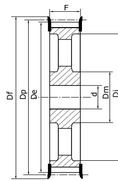
Typ 3EF Hohl-Riemenscheibe
