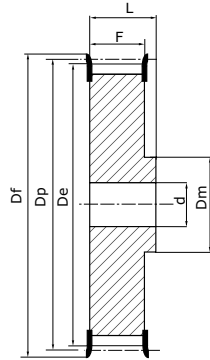
Typ 2F Vollschleibe mit Bordschleiben
