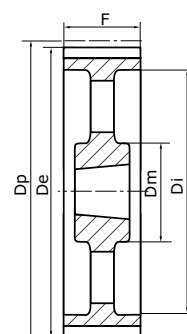
Typ 9E Hohl-Riemenhleibe
