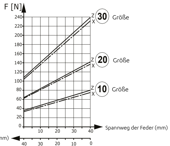
Belastungsdiagramm
