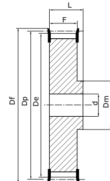
Typ 2F Vollsleibe mit Bordsleiben
