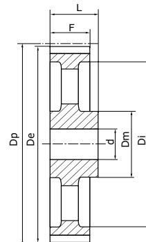
Typ 2E Hohl-Riemenleibe
