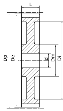
Typ 3A Riemenscheibe
