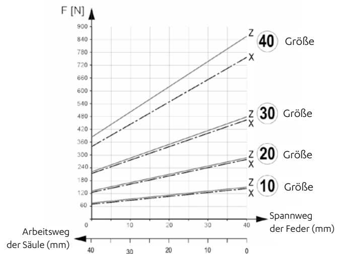
Belastungsdiagramm
