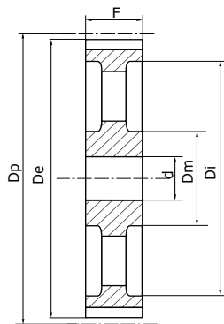
Typ 3E Hohl-Riemenscheibe
